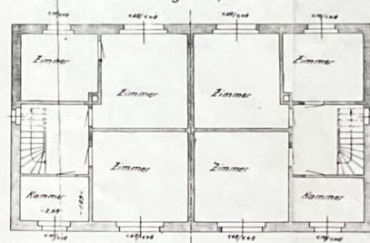
Obergeschoß.
