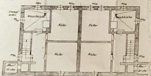
Kellergechoß.
